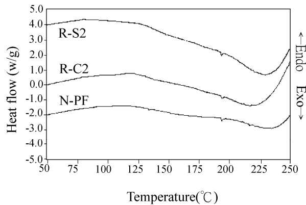
圖 1. Novolak 型酚樹脂之 DSC 熱分析圖
