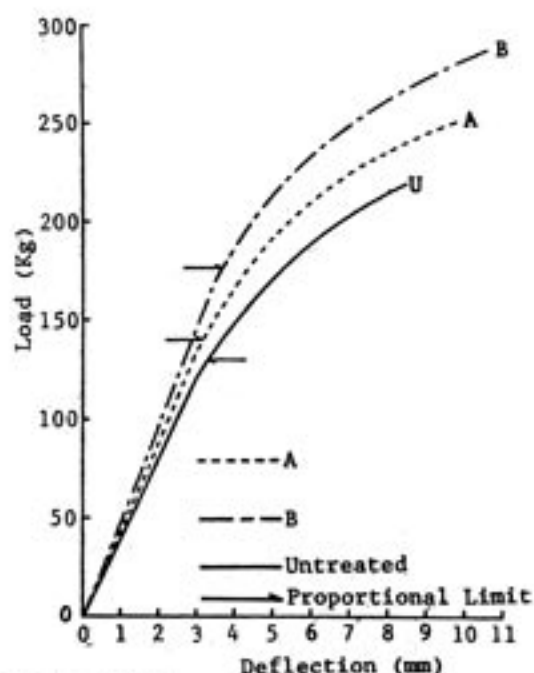
圖 2： 木麻黃抗彎強度之荷重變形圖
